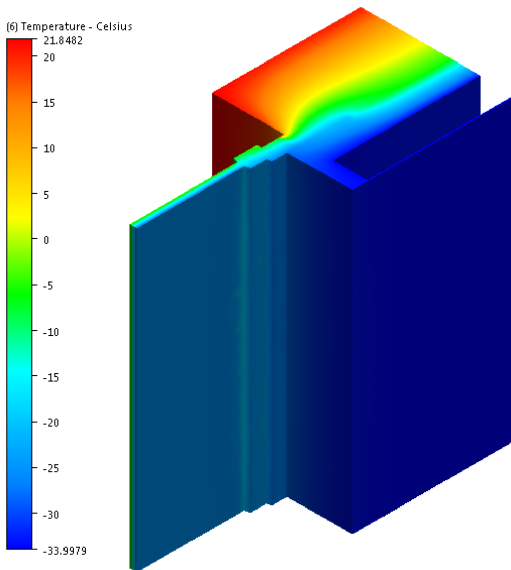
Рисунок 4. Температурные поля откоса из АПКП (разработано автором)
