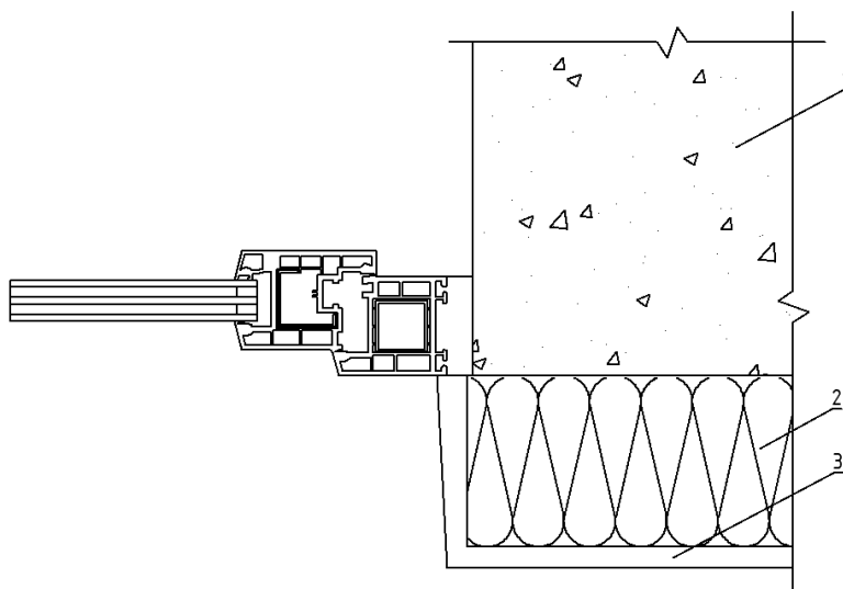
Рисунок 2. Откос с отделкой штукатурным фасадом. 1 – основание; 2 – теплоизоляционная минераловатная плита; 3 – штукатурка (разработано автором)
