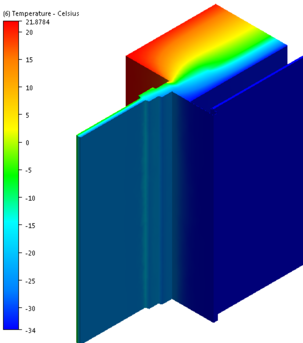
Рисунок 3. Температурные поля откоса из оцинкованной стали (разработано автором)
