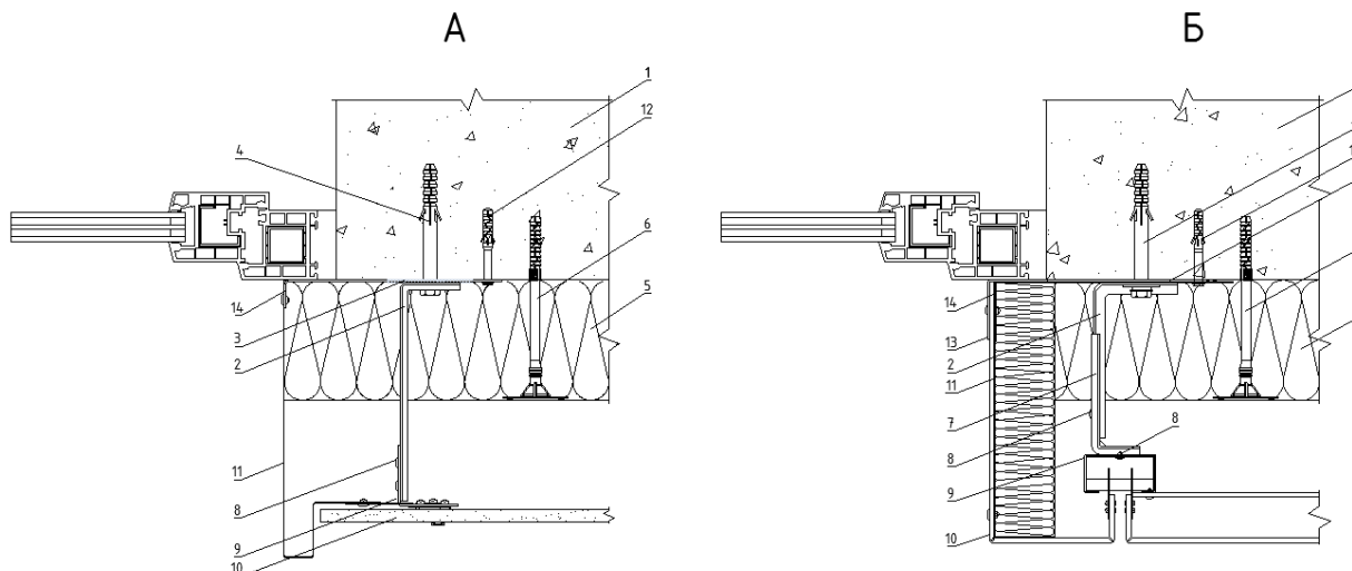
Рисунок 1. Схемы оконных откосов: А – откос из оцинкованной стали; Б – откос из АПКП.
