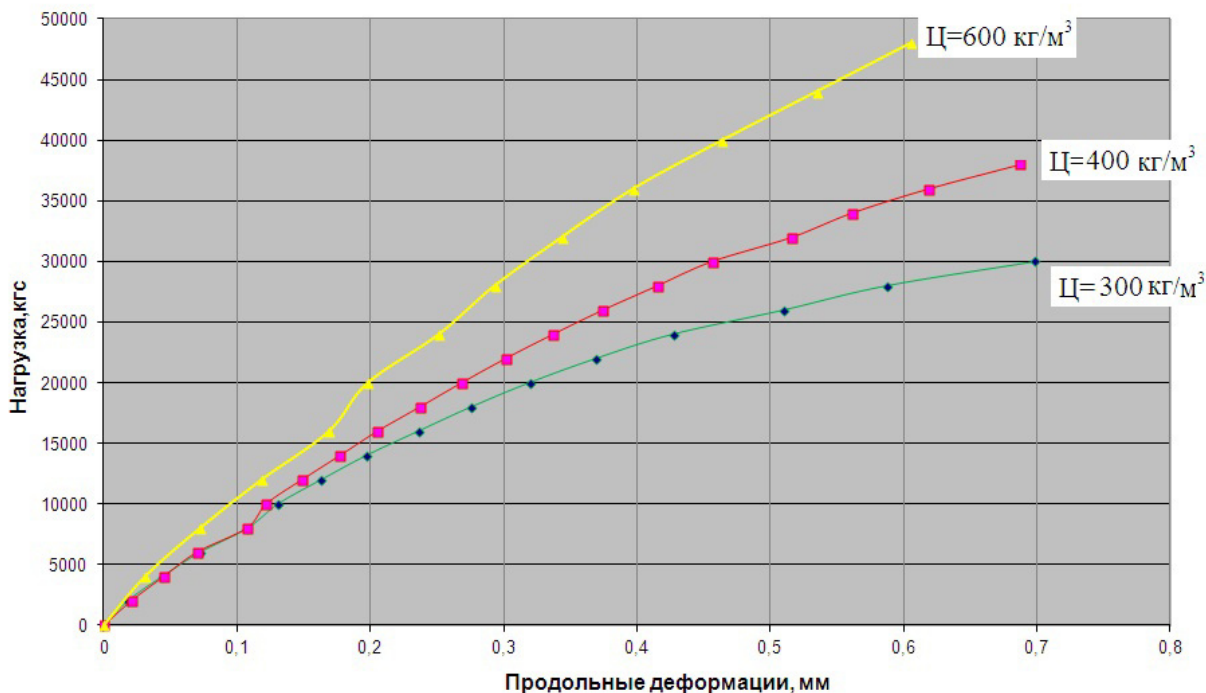
Рис. 2. Зависимость продольных деформаций ЛСУБ при сжатии образцов-призм от величины действующей нагрузки
