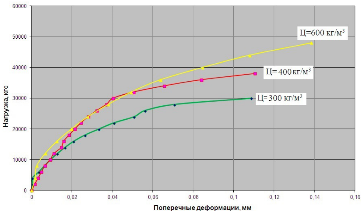
Рис. 3. Зависимость поперечных деформаций ЛСУБ при сжатии образцов-призм от величины действующей нагрузки
