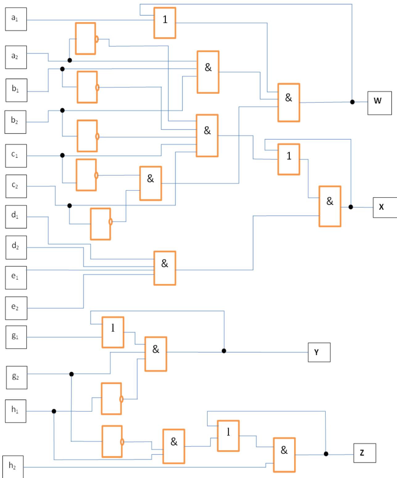
Рис. 4. Функциональная схема УЛУ (разработано авторами)
