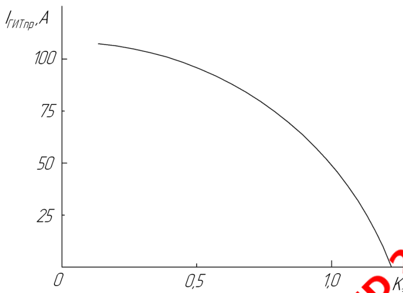
Рис.4.3. Зависимости допустимых значений ГИТ при различной нагрузке силовых трансформаторов ТДЦ-400000/220
